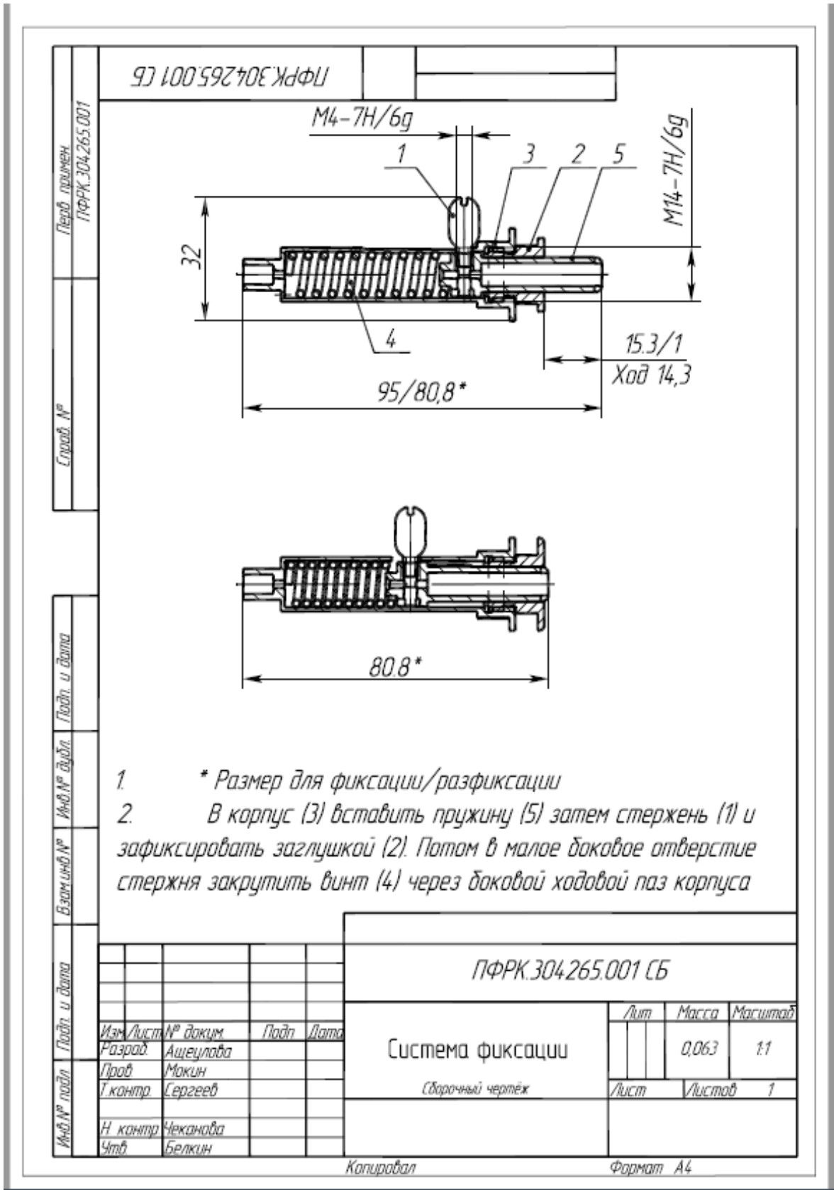
Пример Сборочные чертеж
