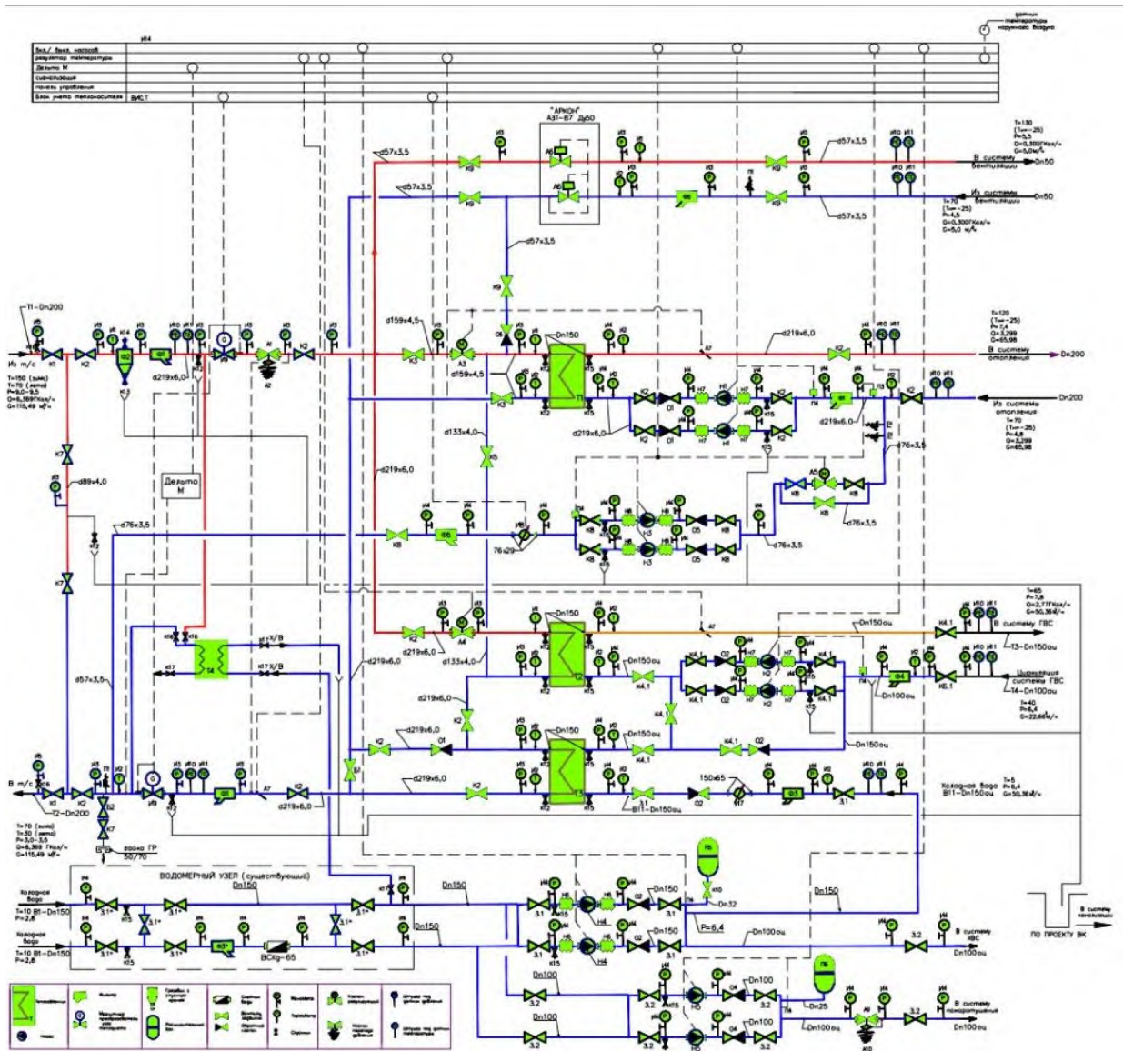
Рис. 1. Проект ИТП
