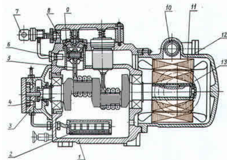
Рис. 1. Поршневой одноступенчатый компрессор марки ПБ-220:
