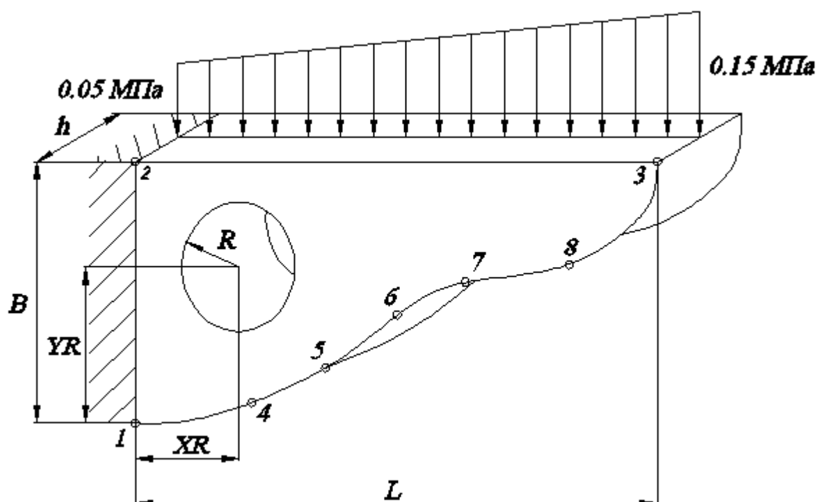
Рис. 1. Чертеж кронштейна
