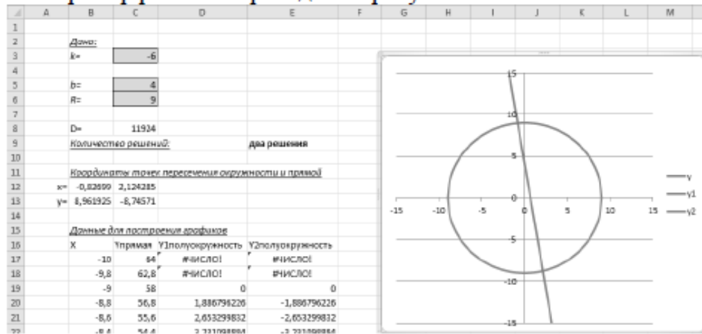
Рис.8.4. Решение задачи пересечения окружности и прямой
