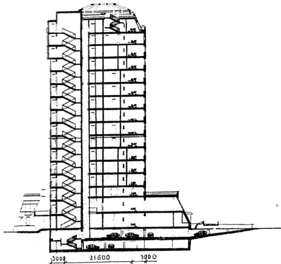
Разрез 1-1
