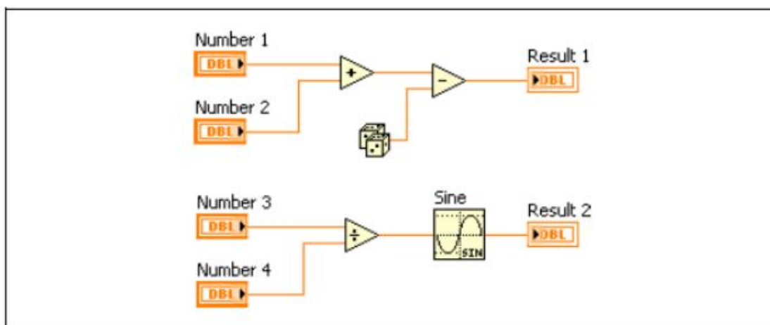
Рисунок 3 – Блок-диаграмма LabVIEW
