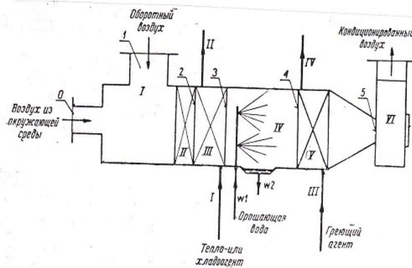
Схема кондиционирующего оборудования. I — смесительная камера; II — фильтр; III — предварительный теплообменник; IV — камера орошения; V — концевой теплообменник; VI — вентилятор.
