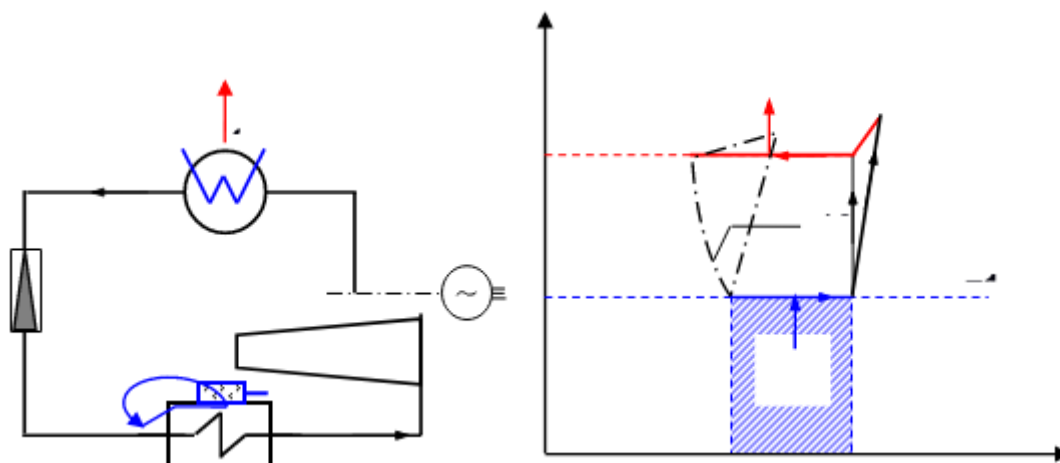
Парокомпрессионная холодильная установка
