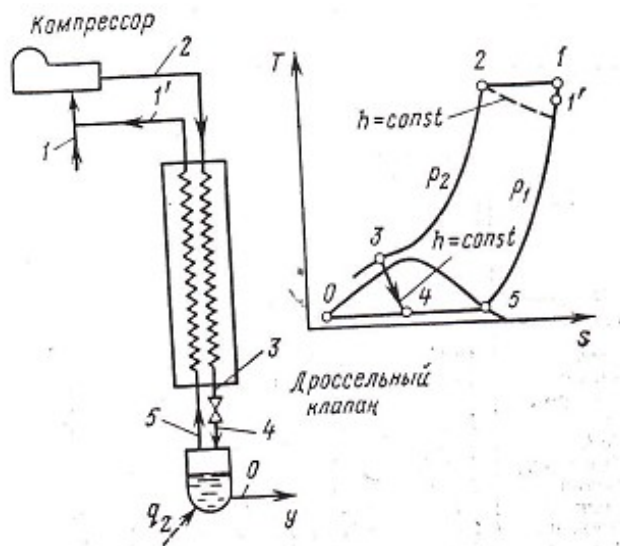
Рис. 3.4. Схема цикла с однократным дросселированием
