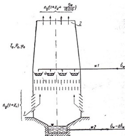
Схема градирни.
