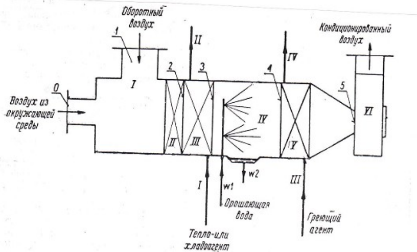
Схема кондиционирующего оборудования. I — смешивательная камера; II — фильтр; III — предварительный теплообменник; IV — камера орошения; V — конечный теплообменник; VI — вентилятор.
