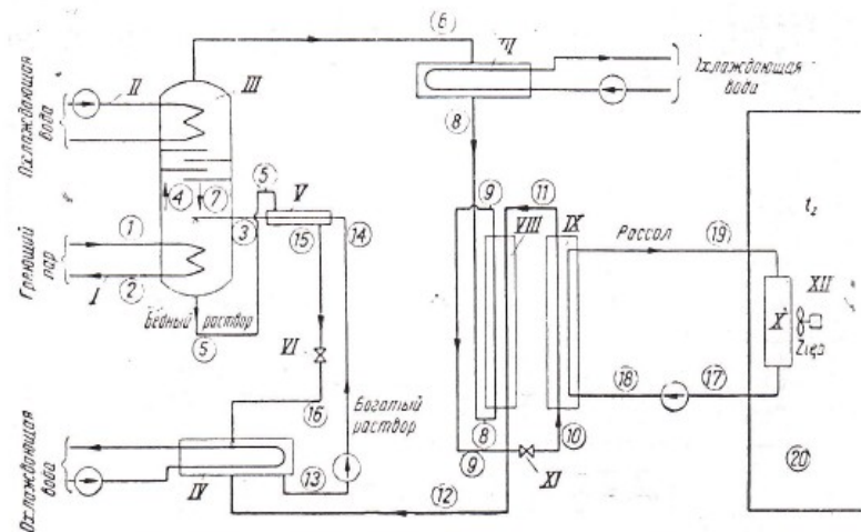
Схема одноступенчатой абсорбционной холодильной установки. I — генератор; II — дефлегматор; III — ректификатор; IV — абсорбер; V — теплообменник; VI — дроссельный вентиль раствора; VII — конденсатор; VIII — охладитель; IX — испаритель; X — нагреватель рассола; XI — дроссельный вентиль хладагента; XII — холодильная камера.
