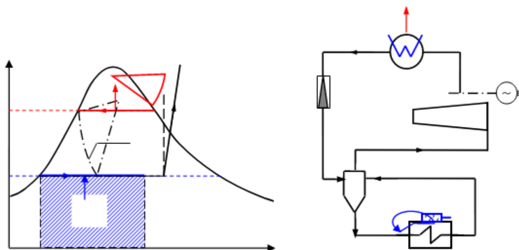
Парокомпрессионная холодильная установка с сепаратором:
