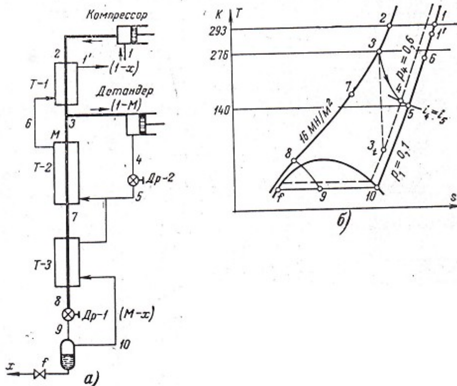
Схема цикла (а) и изображение процессов на диаграмме T-s (б).
