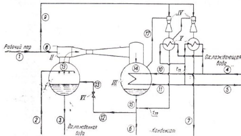
Схема пароэжекторной холодильной установки. I — испаритель; II — основной эжектор; III — основной конденсатор; IV — вспомогательные эжекторы; V — вспомогательные конденсаторы; VI — дроссельный вентиль.
