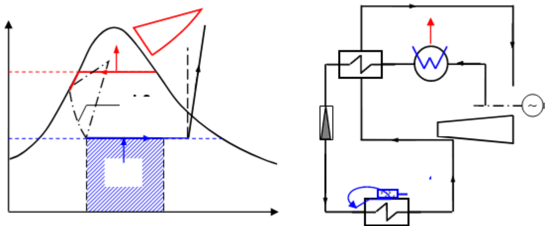
Рис. Парокомпрессионная холодильная установка с регенерацией: а – цикл в T,s- диаграмме; б – схема
