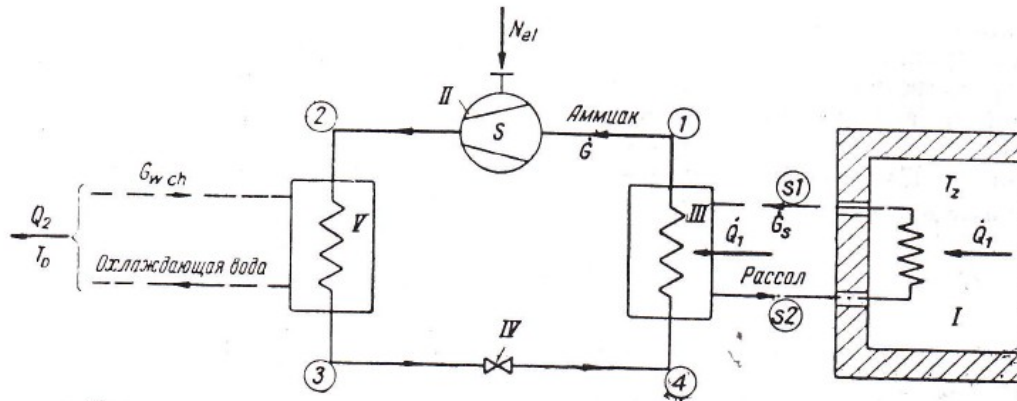
Схема компрессионной холодильной установки. I — холодильная камера; II — компрессор; III — испаритель; IV — регулирующий вентиль; V — конденсатор.
