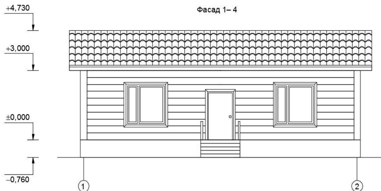
Рисунок 2.2 - Фасад книгохранилища
