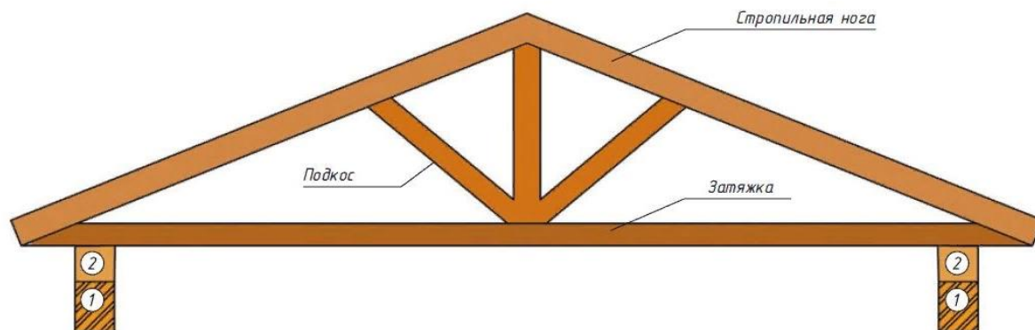
Рисунок 4.8 - Схема стропильной системы
