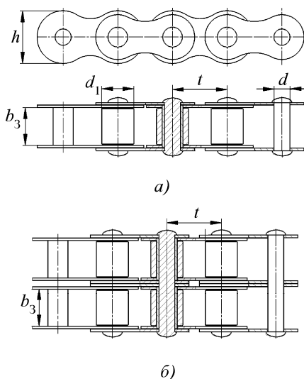
Рис. 10.2. Цепь роликовая:
