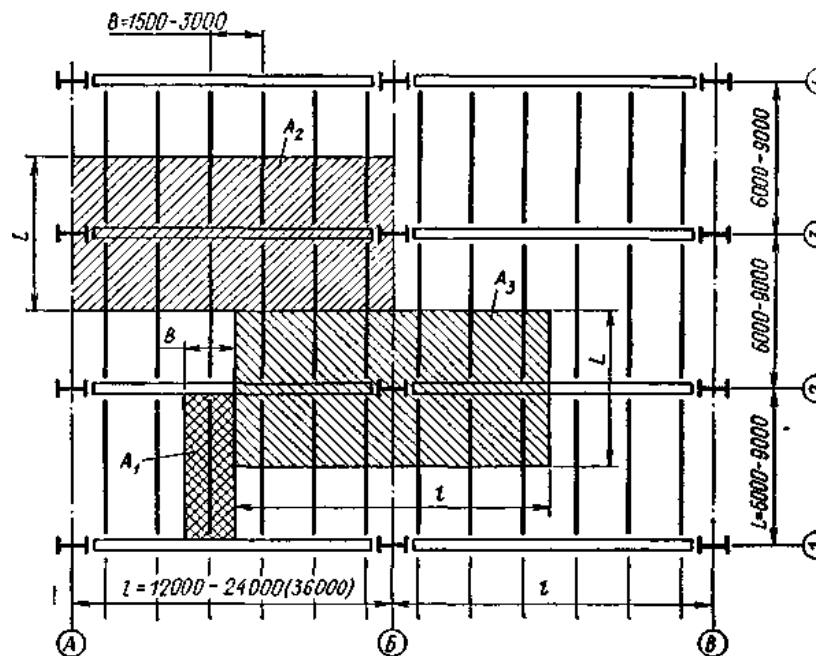
Рис. 1. Балочная клетка:
