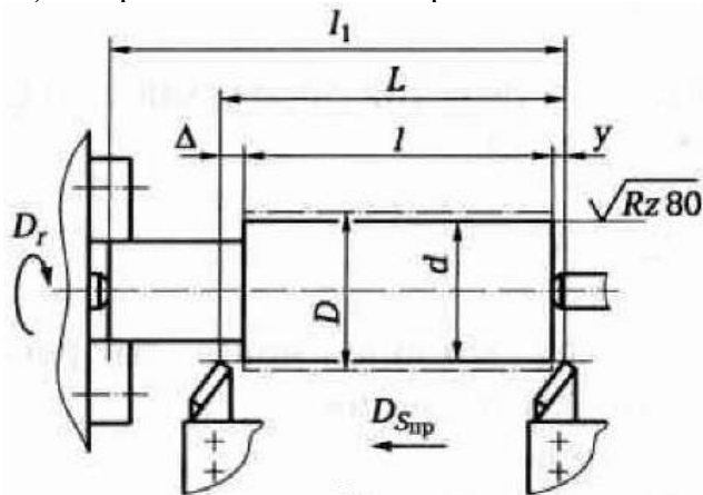
Рис. 1. Эскиз обработки
