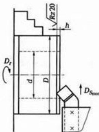
Рис. 2. Эскиз обработки
