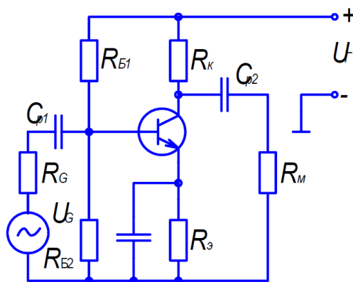
Рис 1 Принципиальная электрическая схема усилительного каскада
