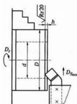
Рис. 2. Эскиз обработки
