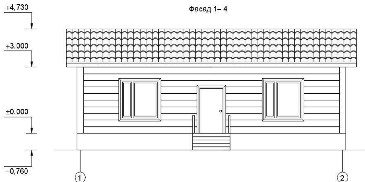
Рисунок 2.2 - Фасад книгохранилища
