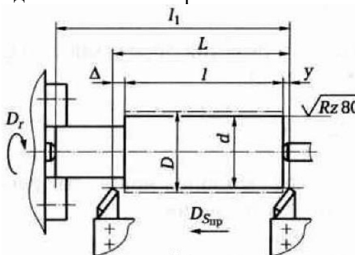
Рис. 1. Эскиз обработки
