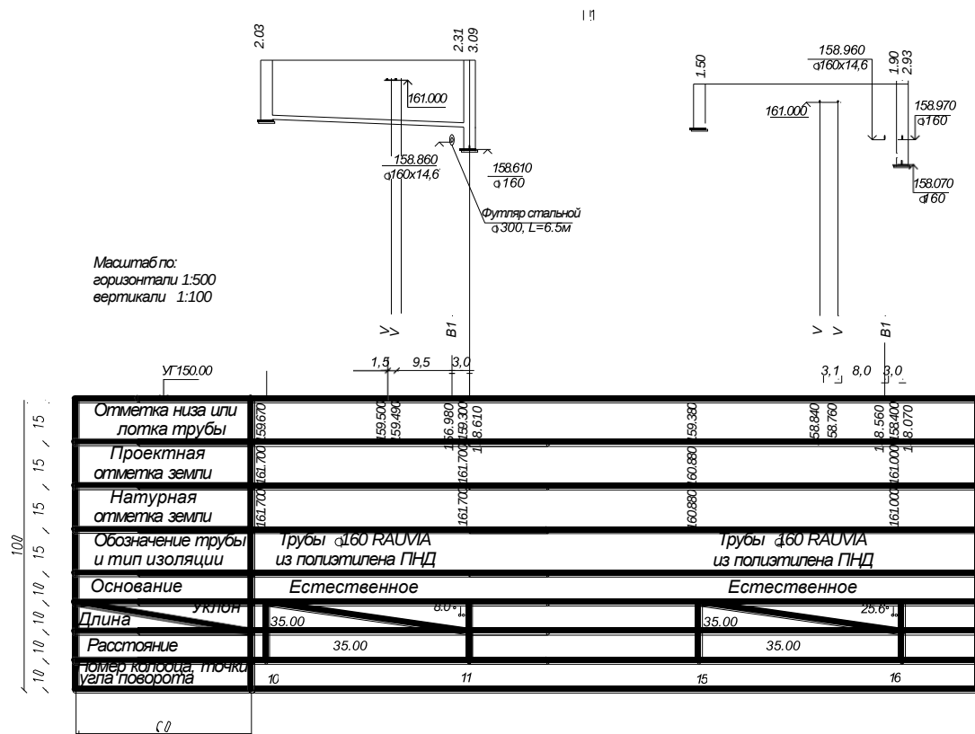
Рис.5.5. Пример построения продольного профиля дворовой канализационной сети
