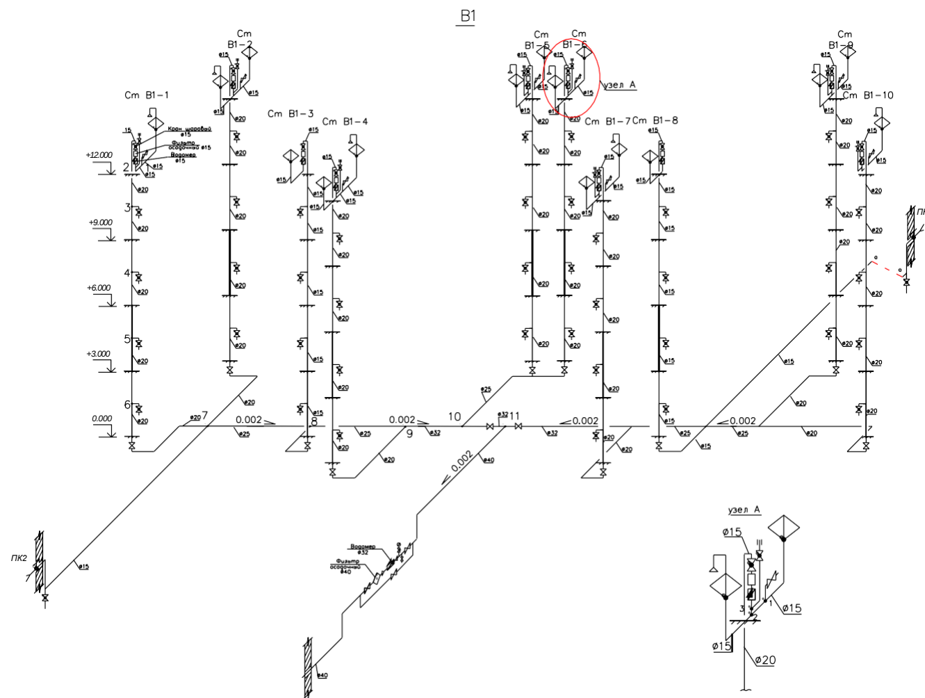
Рис.5.1. Аксонометрическая схема внутреннего водопровода
