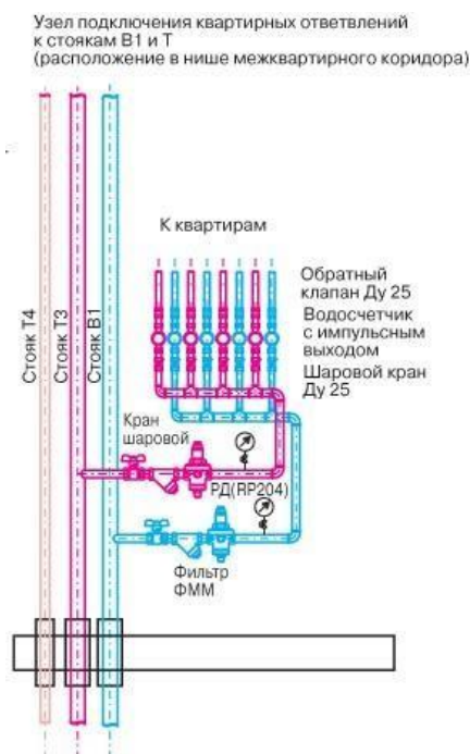
Рис. 1. Схема поэтажного коллекторного присоединения квартирных трубопроводов В1, Т3, Т4 к стоякам, расположенным в нишах межквартирных коридоров
