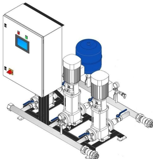
Рис. 3. Повысительная насосная установка с тремя вертикальными насосами и гидропневматическим баком
