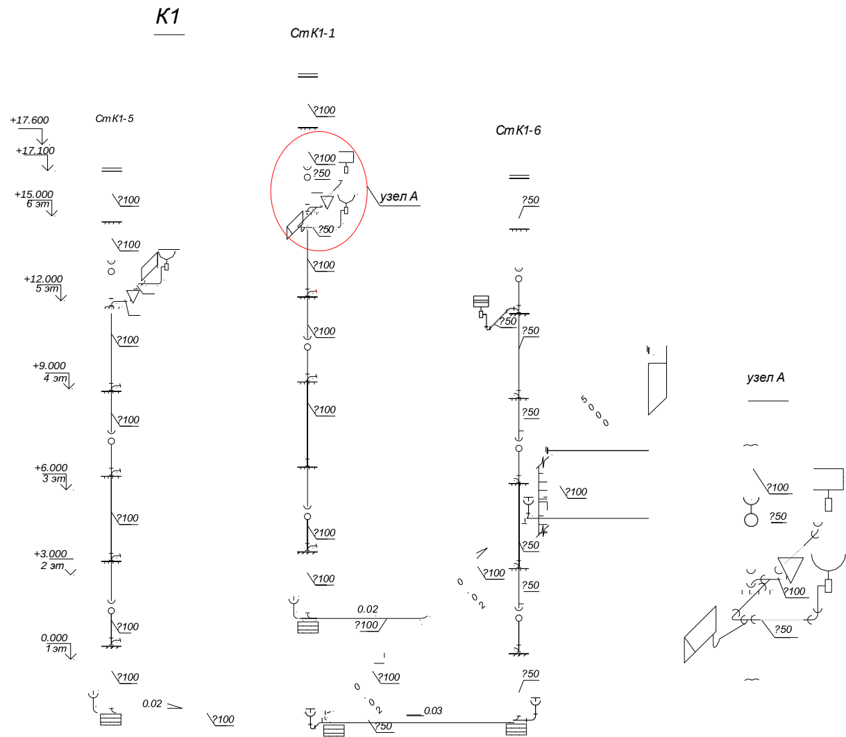
Рис.5.2. Аксонометрическая схема трубопроводов канализационных стояков и выпуска
