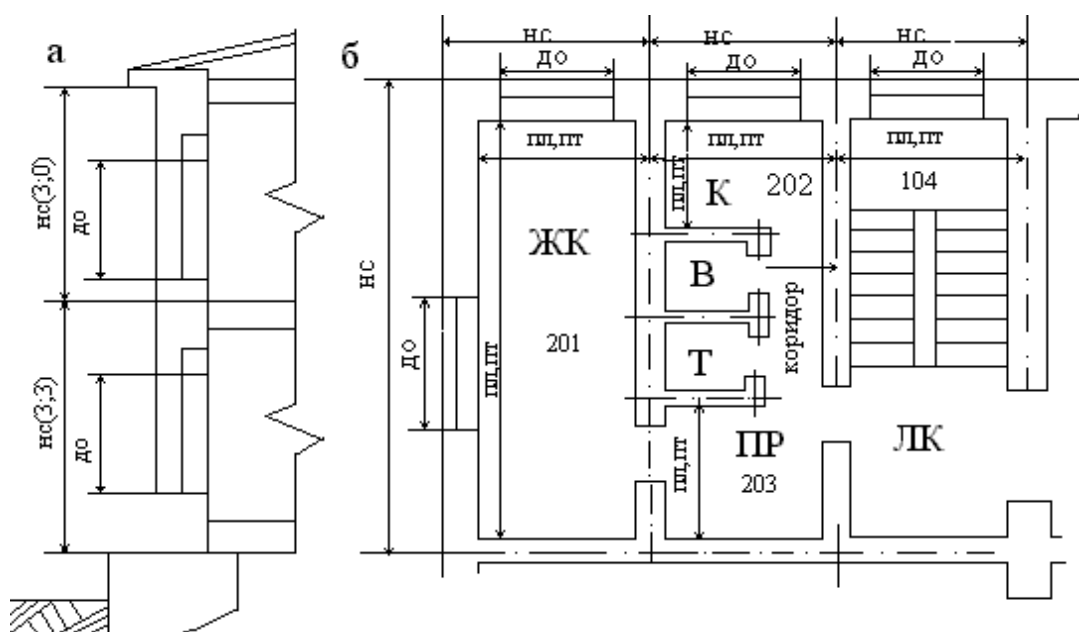
Рис. 3.1. Схема обмера ограждающих конструкций (размеры в м):
