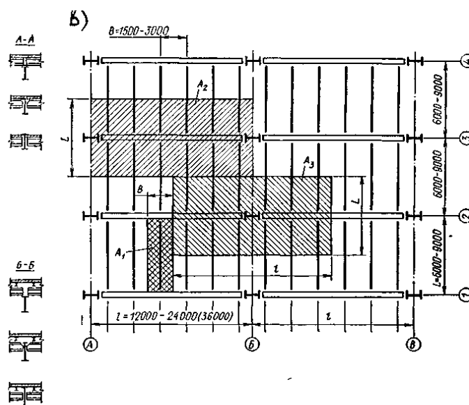
Рис. 2.1. Балочная клетка:
