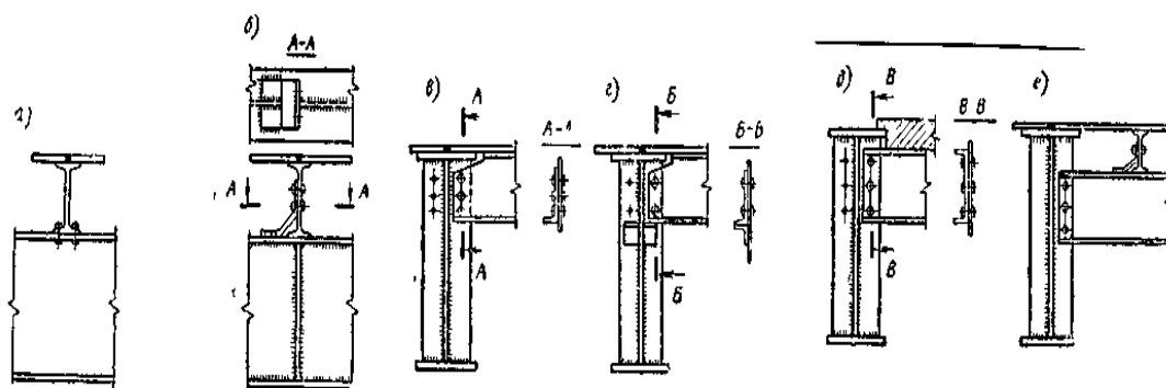
Рис. 2.4. Виды спряжения балок настила, второстепенных и главных балок:
