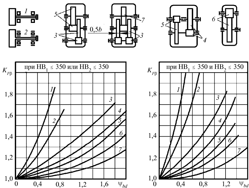
Рис. 8.12. Графики для определения коэффициента K_{Fp}
