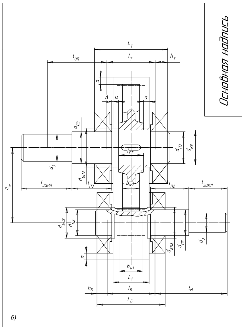
Рис. 12.8. Продолжение
