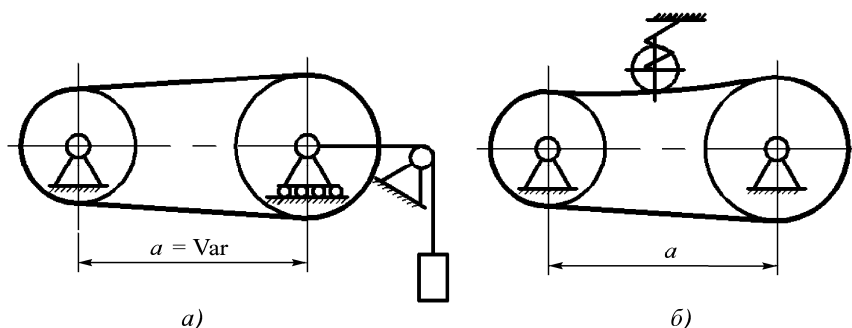
Рис. 11.4. Передачи с автоматическим натяжением ремня (I группа): a – грузовое натяжение; б – натяжение роликом
