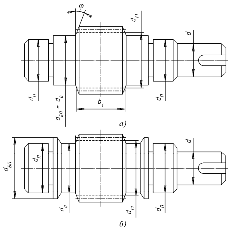
Рис. 12.5. Конструкции червяков:
