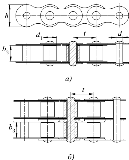
Рис. 10.2. Цепь роликовая:
