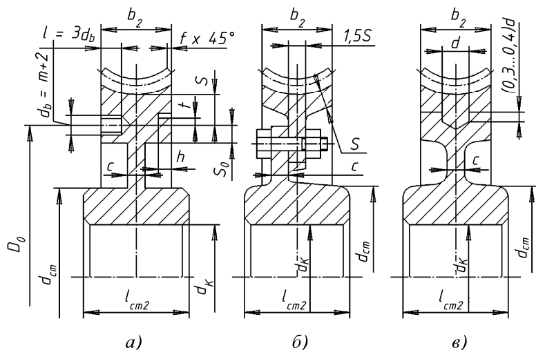
Рис. 12.6. Конструкции составных червячных колес, образованных соединением зубчатого венца с центром:
