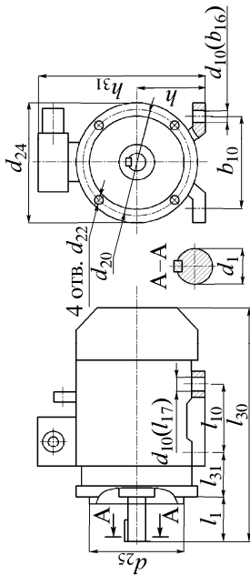
А3. Габаритные, установочные и присоединительные размеры двигателей серии АИР исполнения М2081 (М2082)
