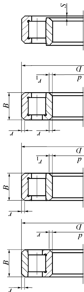
Б9. Подшипники роликовые с короткими цилиндрическими роликами (ГОСТ 8328-75)
