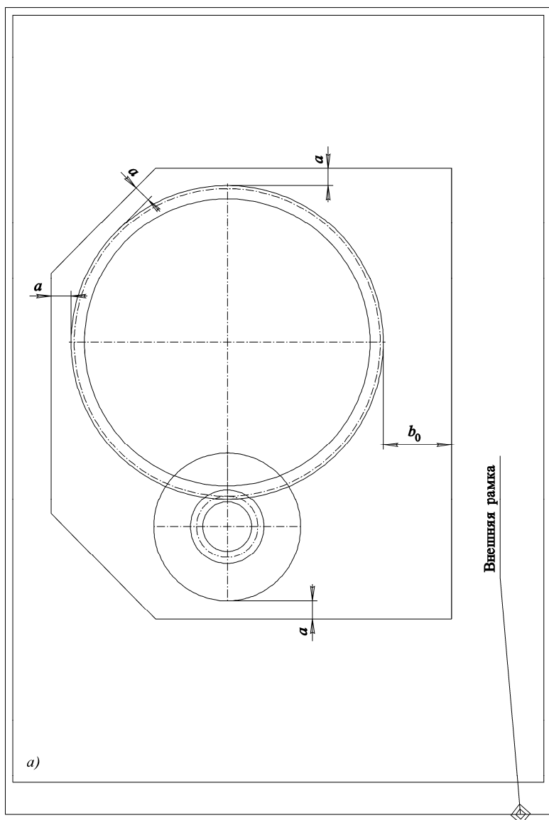
Рис. 12.8. Пример эскизной компоновки зубчатого цилиндрического одноступенчатого редуктора: a – главный вид; б – вид сверху
