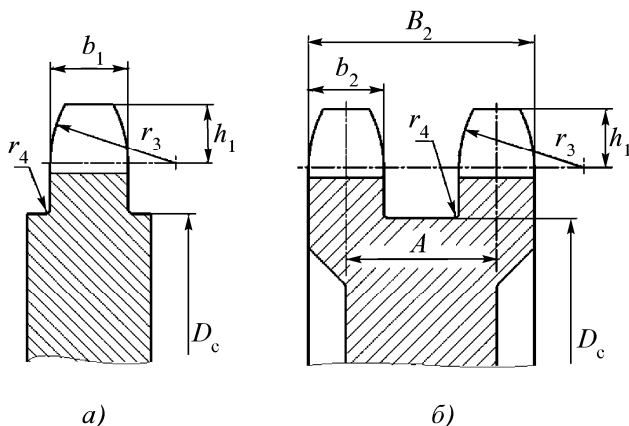
Рис. 10.4. Звездочки для передач:
