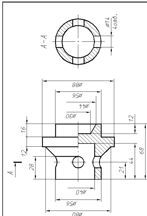
Вентиль
