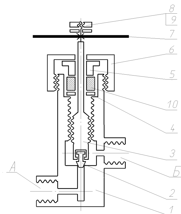
Клапан 803.002
