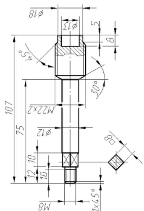
Шпиндель 803.003
