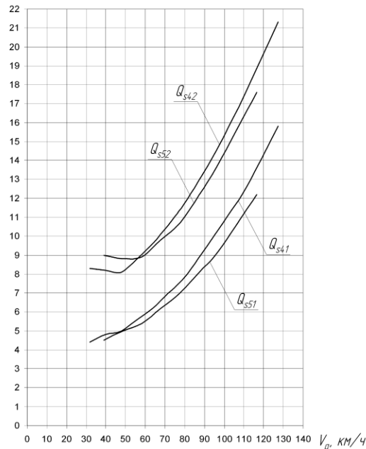
Экономическая характеристика автомобиля
