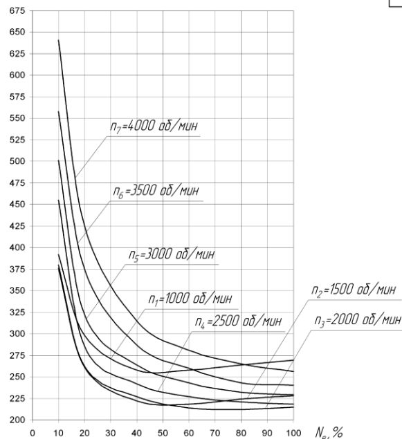
Нагрузочная характеристика двигателя
