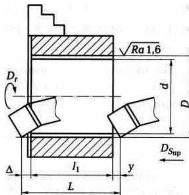
Рис. 3. Эскиз обработки
