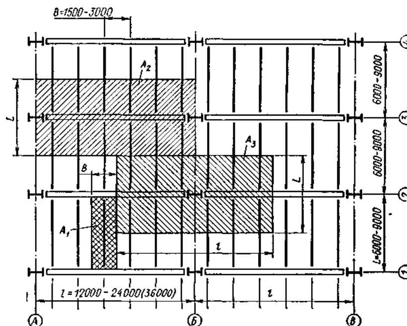
Рис. 1. Балочная клетка:
