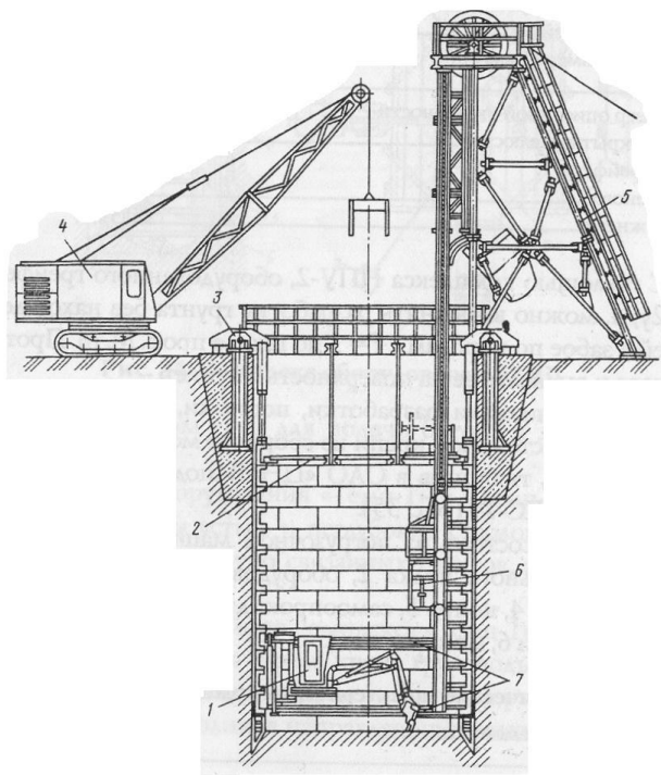
1 - погрузочная машина; 2 - подвесной предохранительный полок; 3 - оборудование для задавливания крепи; 4 - кран; 5 - копёр; 6 - самопрокидная скипоклеть или опрокидная клеть; 7 - монорельс.
