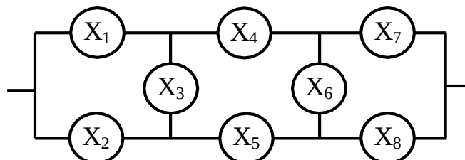
Рис. 5.8. Система со структурной схемой типа «лестница»
