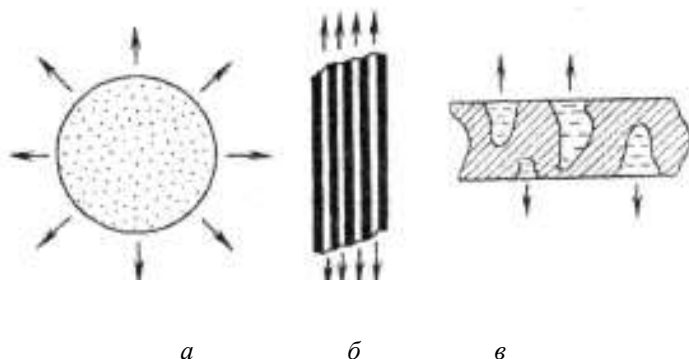
Рисунок 6.8. — Изотропные и анизотропные структуры твердых тел: а — изотропное пористое тело; б — анизотропное пористое тело с регулярной структурой; в — анизотропное пористое тело с нерегулярной структурой
