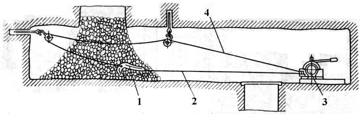
Рис.8.1. Скреперная установка
