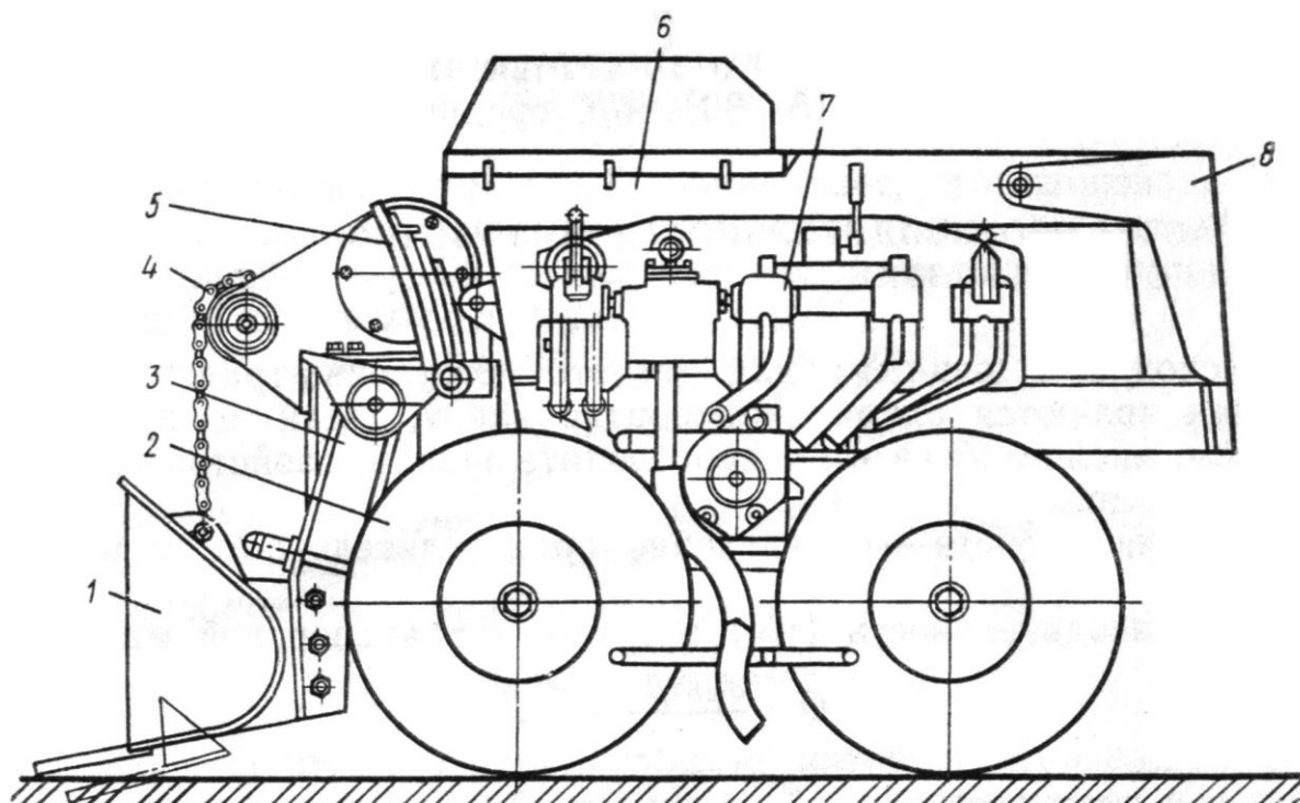
Рис.4.2. Погрузочно-транспортная машина типа ПТ
