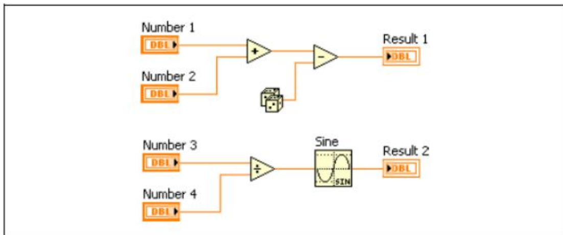
Рисунок 3 – Блок-диаграмма LabVIEW
