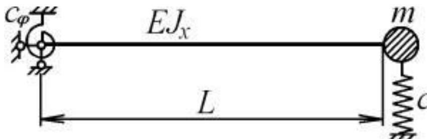
Рис. 1 Расчетная схема
