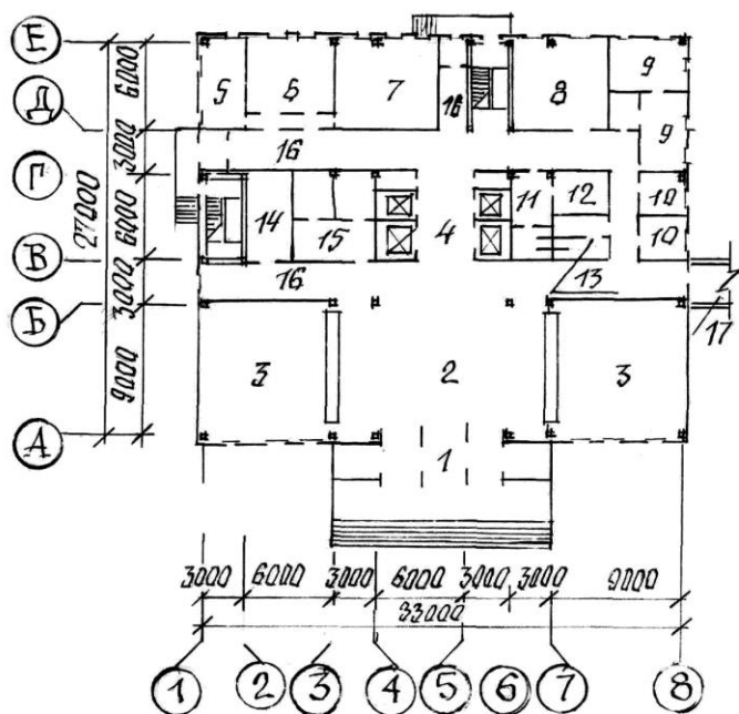
План 1ого этажа
