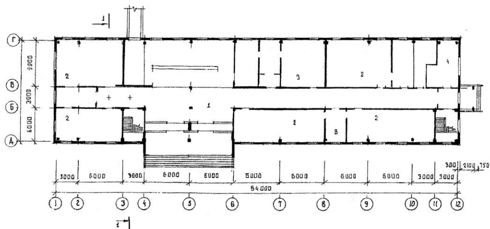
План 1 этажа на отметке 0.00
