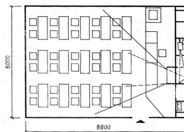
Вариант планировки учебного помещения
