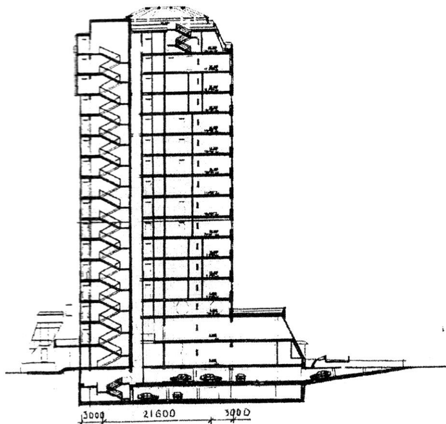
Разрез 1-1
