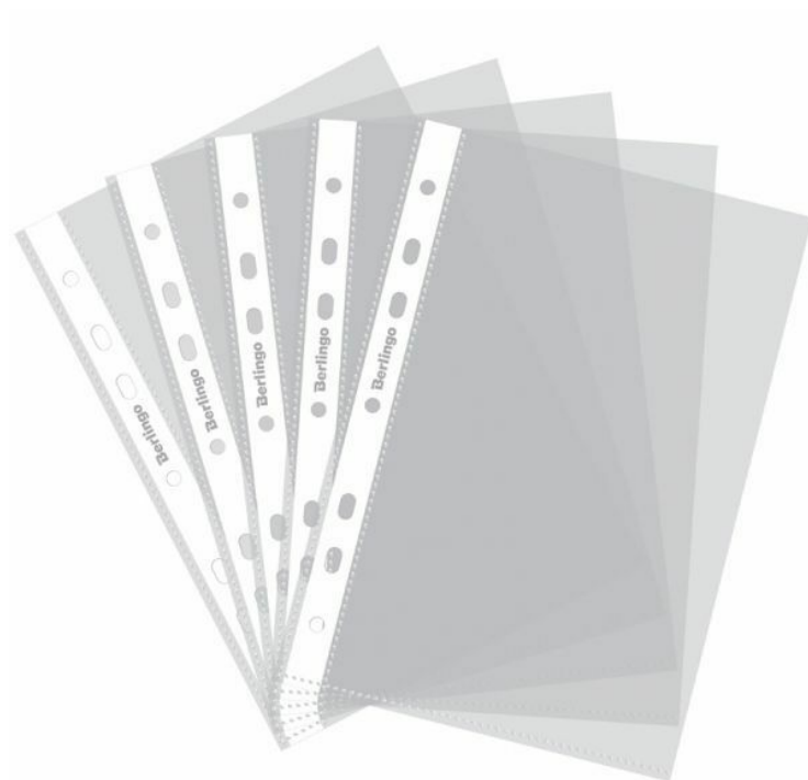
Рисунок 2 — Прозрачные файлы
