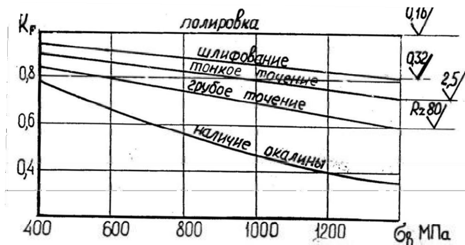
Рис. П.1. Значение коэффициента влияния шероховатости поверхности K_F
