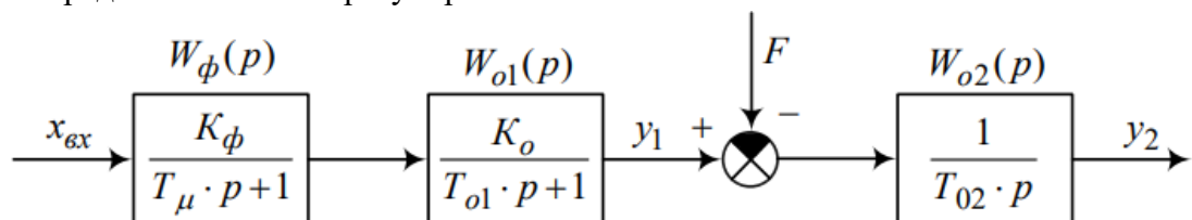
Рис. 1 Объект регулирования
