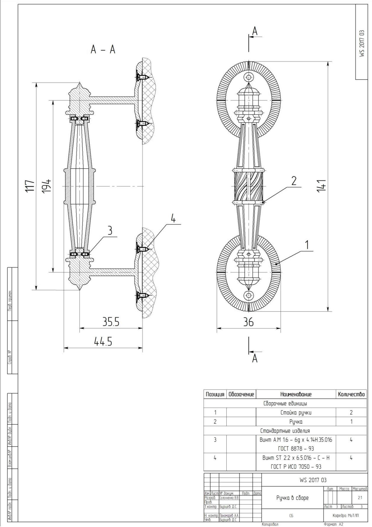
Рисунок 7.Чертёж сборки ручки (М3).
