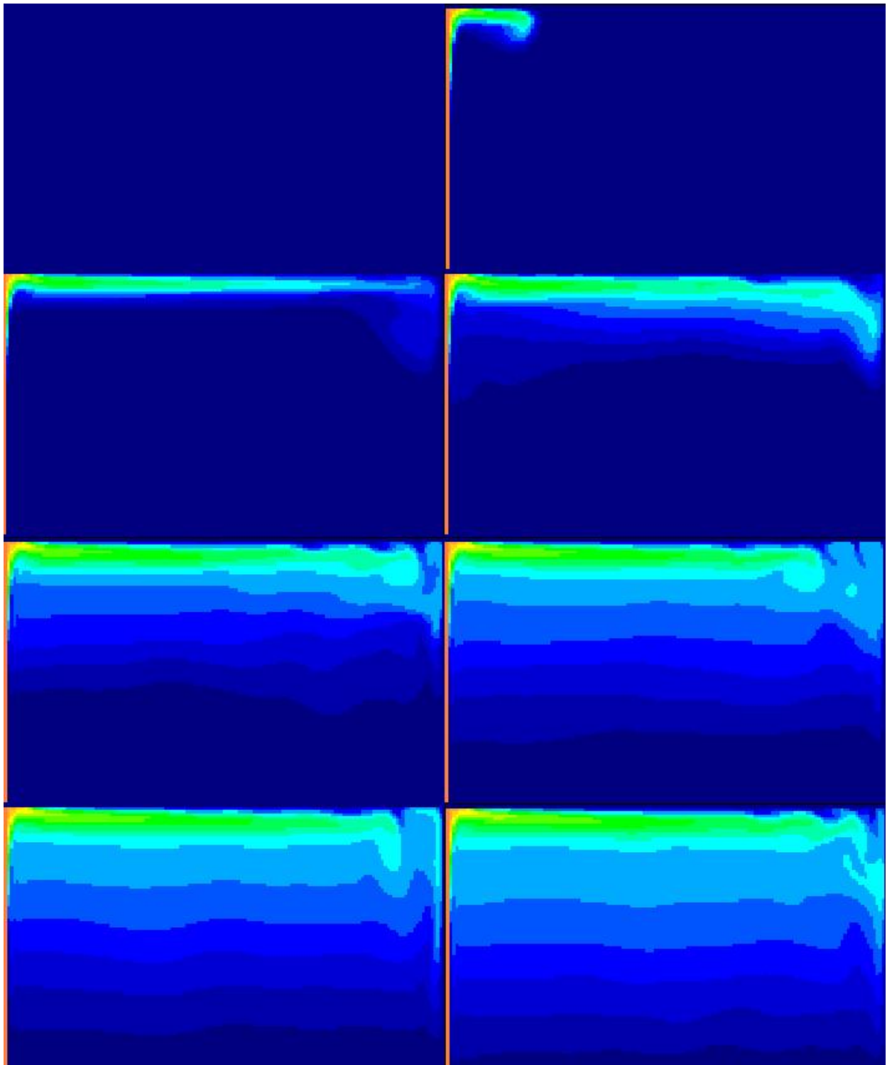
Рис. 3. Нагрев левой стенки ( t = 10 \text{ мин} )
