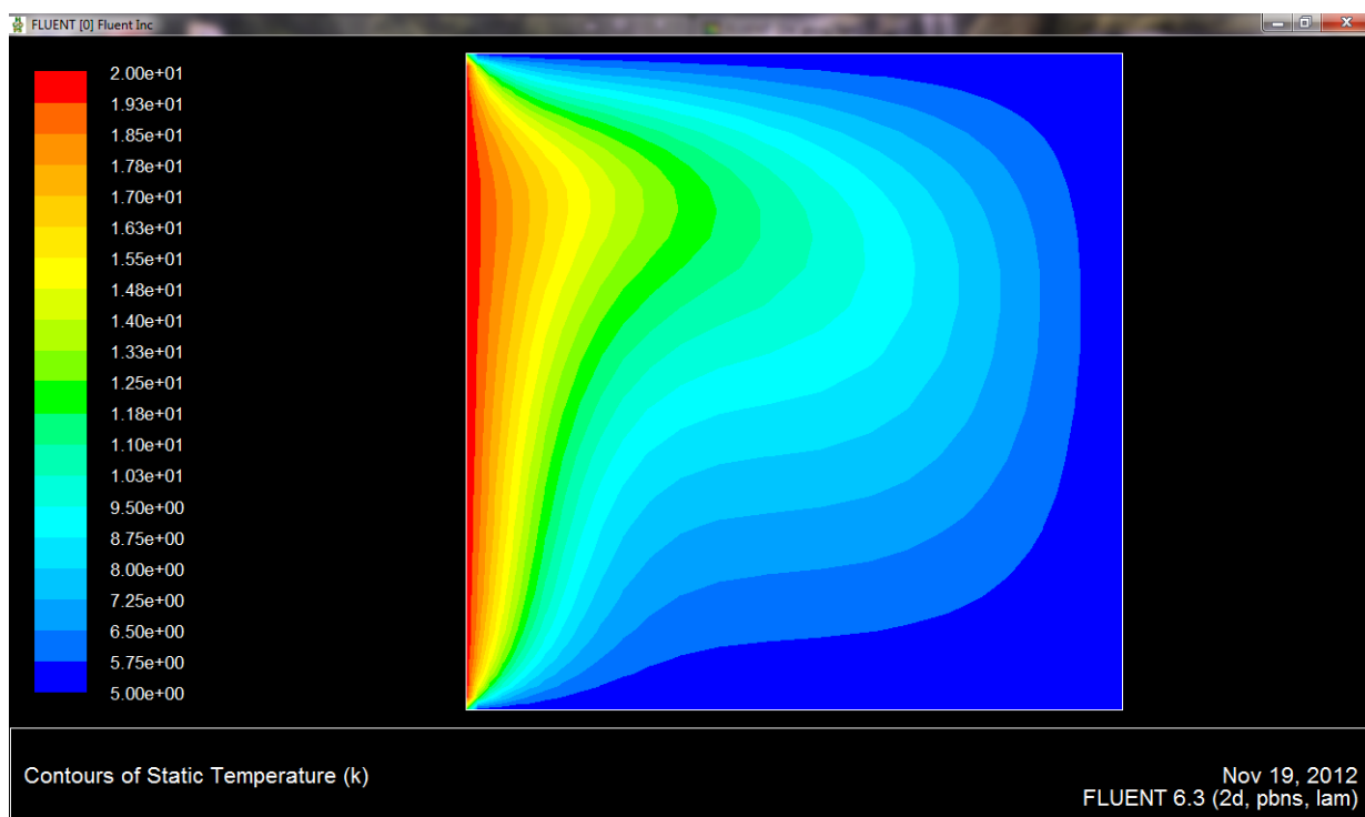
Рис.7. Распределение температуры
