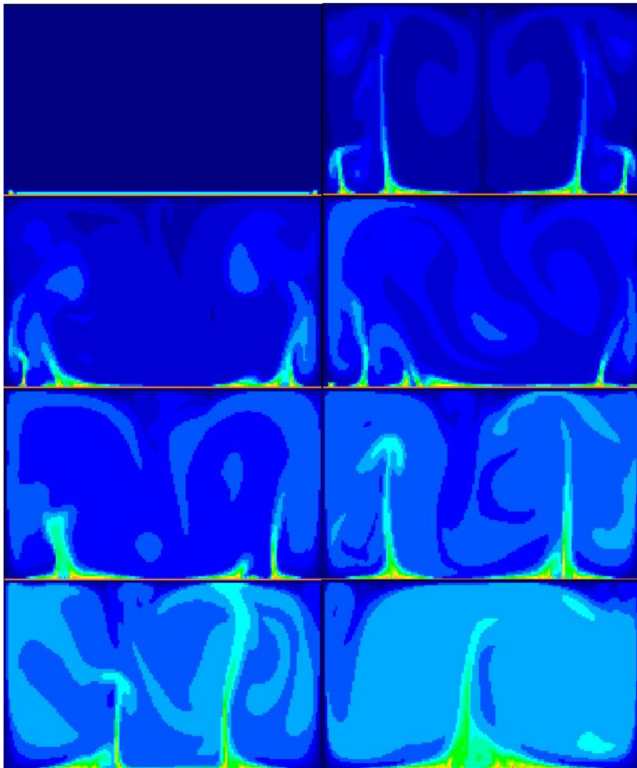
Рис. 2. Нагрев нижней стенки ( t = 10 \text{ мин} )
