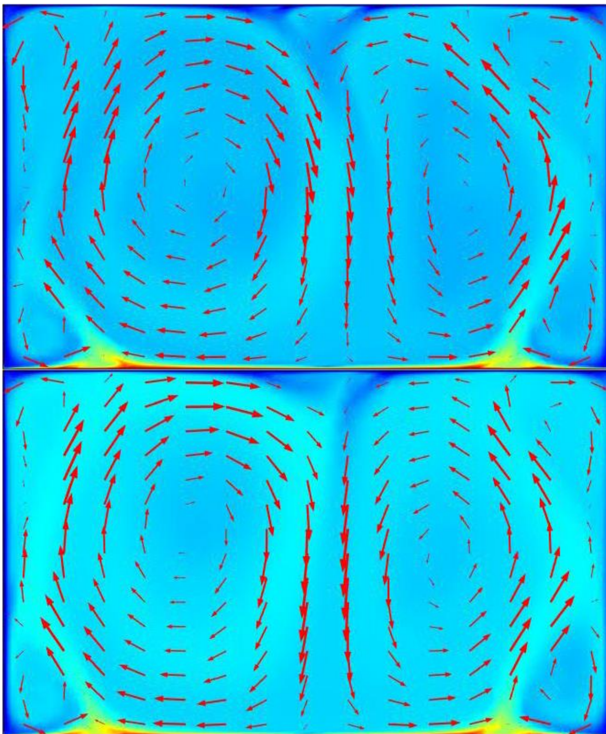
Рис. 9. Нагрев нижней стенки ( t = 10 \text{ мин} )
