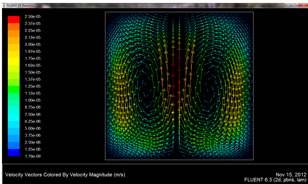
Рис.4. Распределение скоростей
