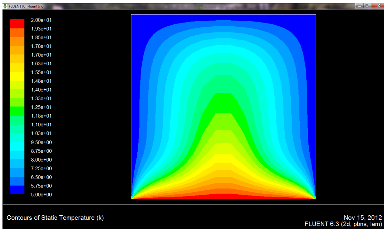
Рис.5. Распределение температуры
