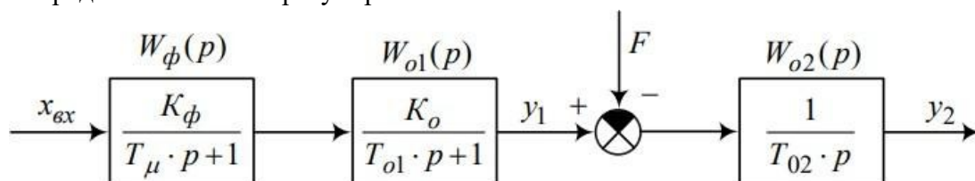
Рис. 1 Объект регулирования
