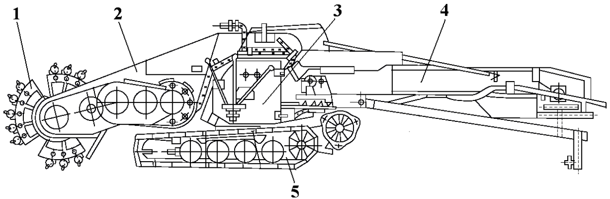
Рис.6.5. Комбайн КДР-6
