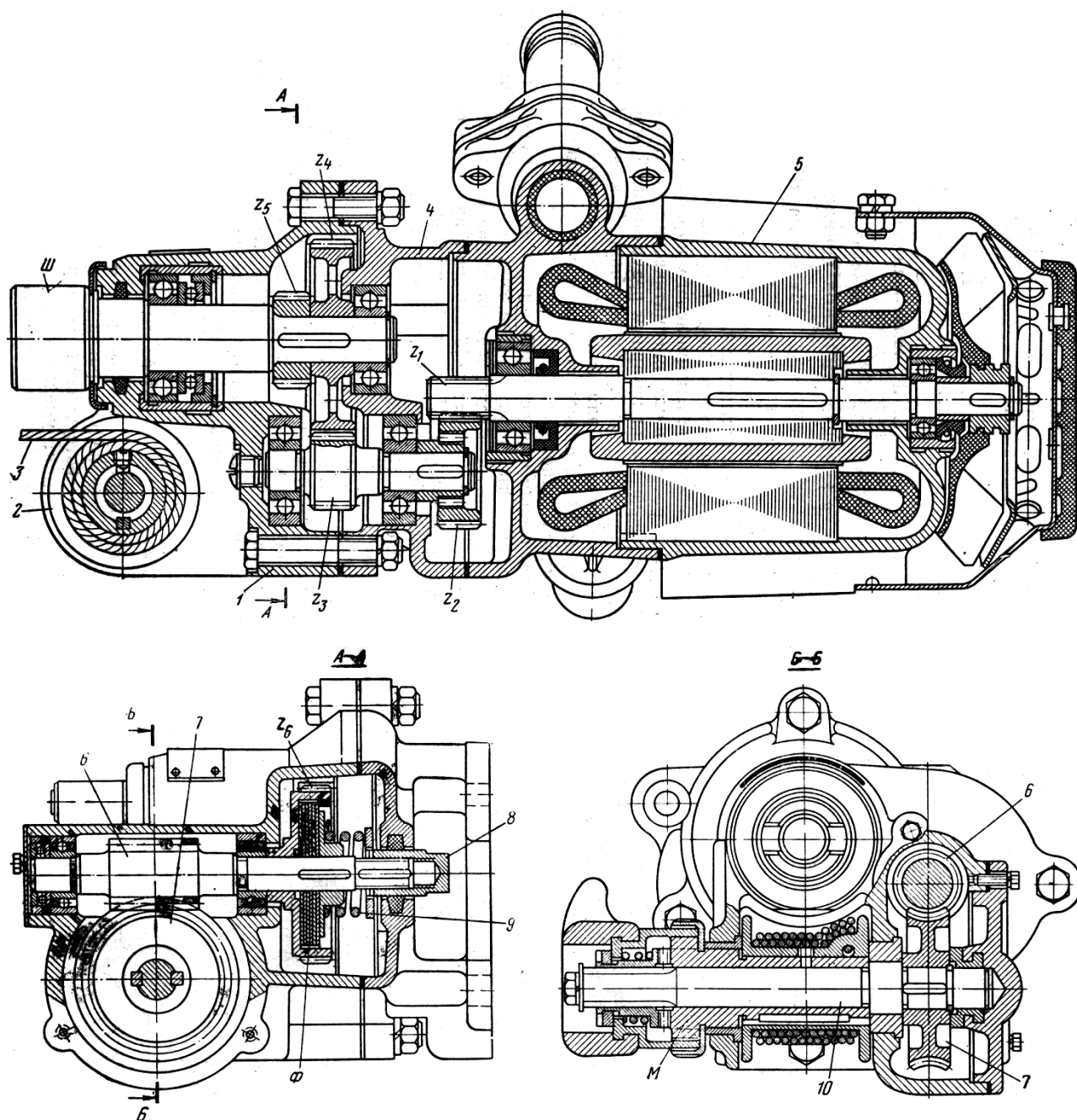
Рис.2.2. Электросверло с принудительной подачей ЭРП-18ДМ
