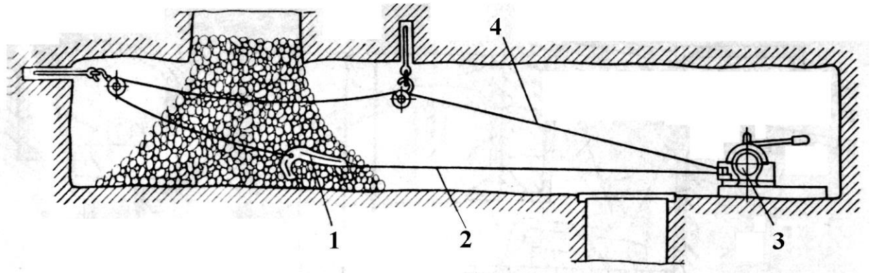
Рис.8.1. Скреперная установка
