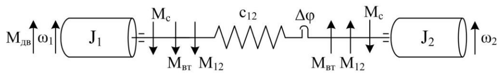
Рисунок Е.1. Кинематическая схема двухмассовой системы
