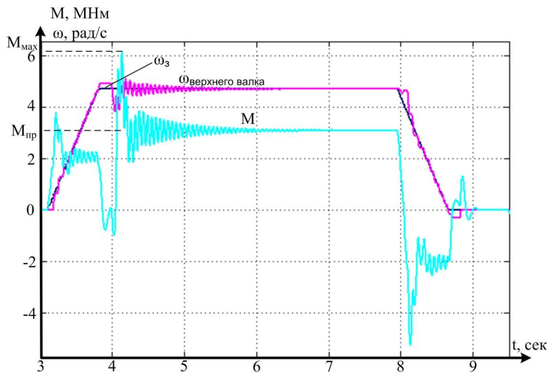
Рисунок Е.2. Переходные процессы момента и скорости электропривода рольганга
