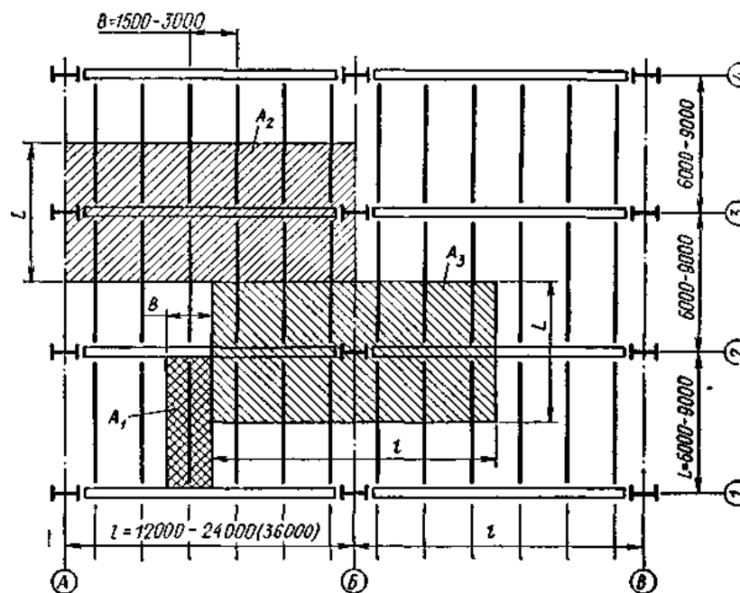
Рис. 1. Балочная клетка:
