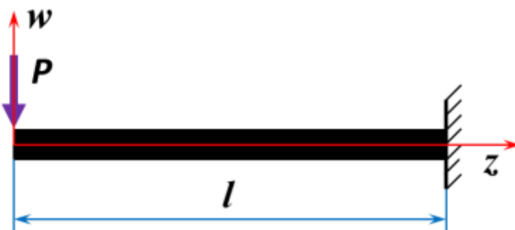
Рис. 1. Расчетная схема
