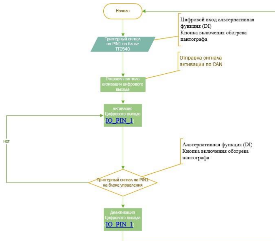
Рисунок 1 – Функциональная блок схема алгоритма управления
