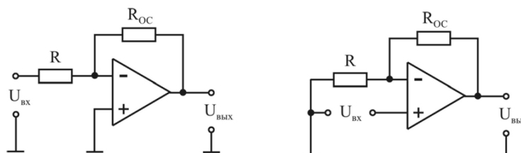
Рис. 4. Инвертирующий и неинвертирующий ОУ
