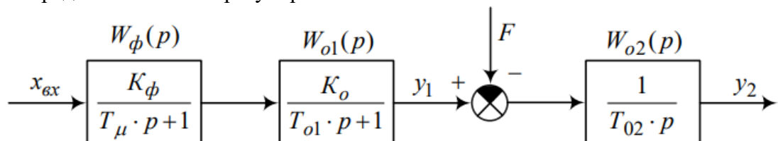
Рис. 1 Объект регулирования
