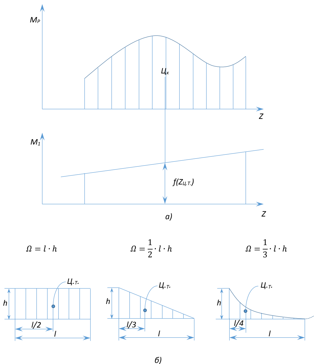
Рис. 3. Схема определения интегрального выражения по способу Верещагина (а) и основные параметры для простейших фигур (б).
