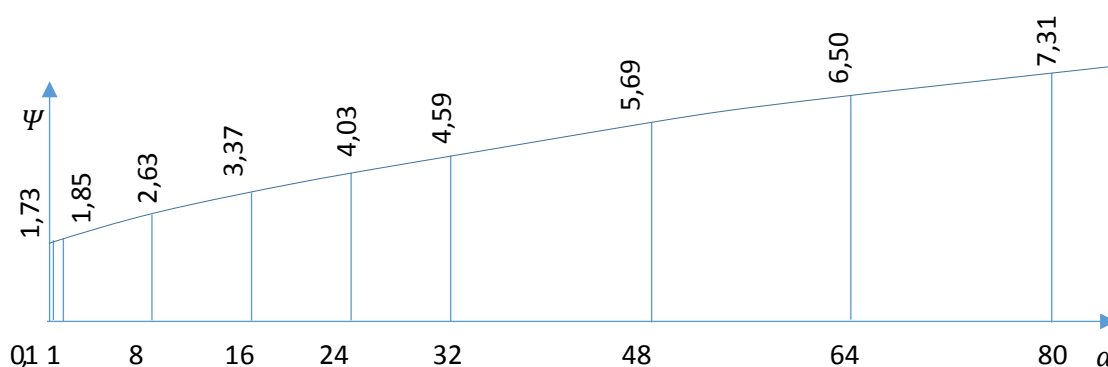
Рис. 6. Функция \Psi(\alpha)
