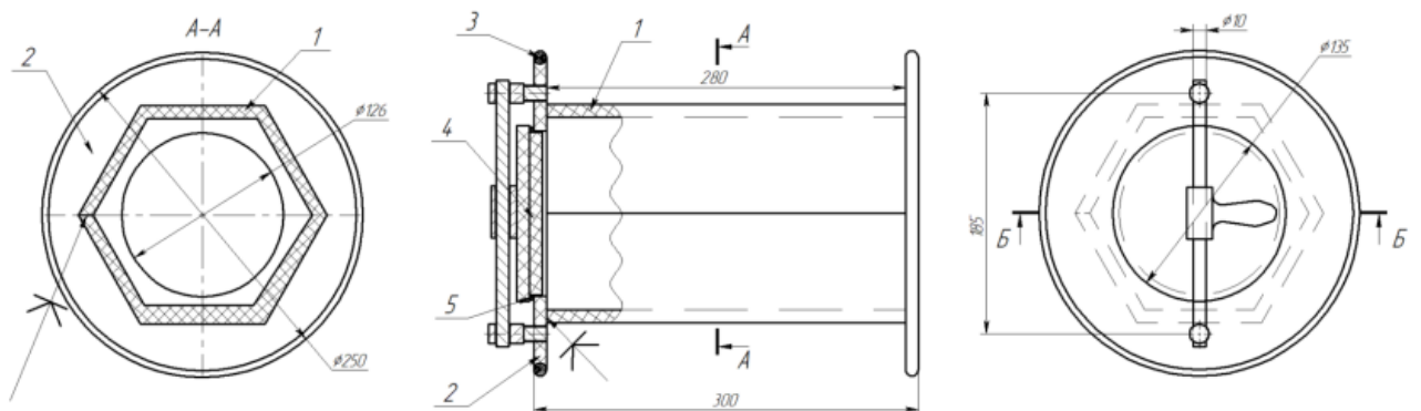
Рисунок 5. Галтовочный барабан.
