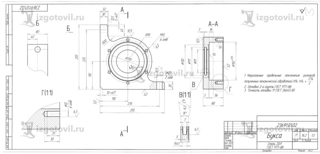
Рисунок 6. Чертёж детали для ЛР4.
