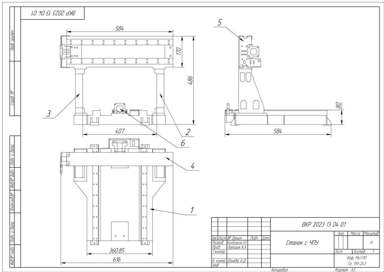
Рисунок 4.2. Чертеж станка с ЧПУ
