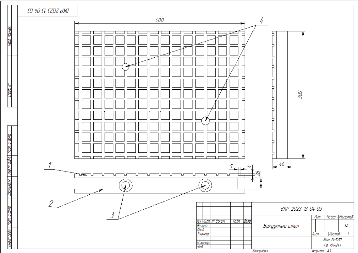
Рисунок 4.4. Вакуумный стол
