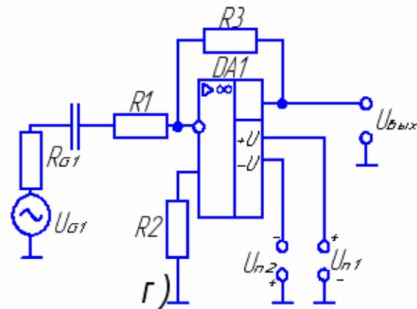
г) инвертирующий усилитель переменного тока
