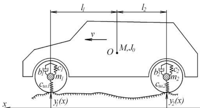
Рис. 1 Схема
