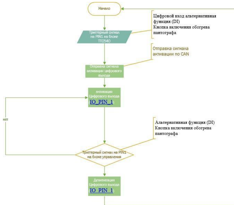
Рисунок 1 – Функциональная блок схема алгоритма управления
